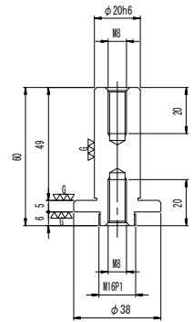
シャックφ20詳細図
