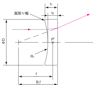
合成石英平凹レンズ
