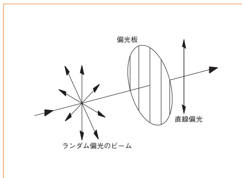
↑ 偏光板
