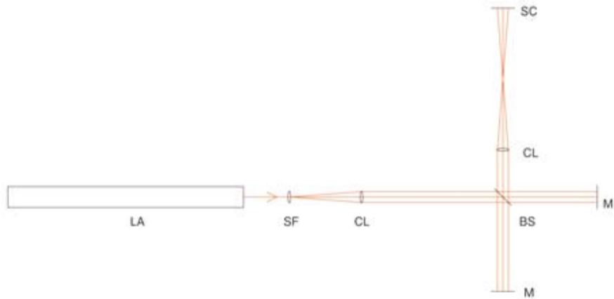
トワイマン・グリーン干渉計 光学系
