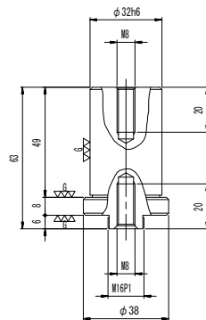
シャックφ32詳細図
