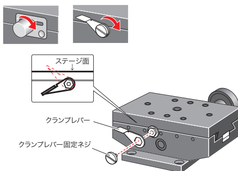
クランプ方式
