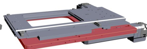
2 軸電動 XY ステージ
