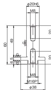
シヤク \phi 20 詳細図
