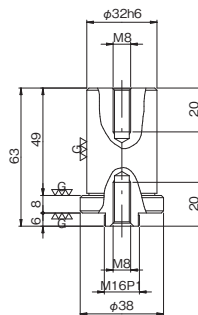
シヤク \phi 32 詳細図
